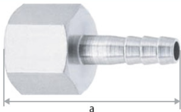
PNEUMATIK IG VPG hadicový trn s vnitřním závitem kód 30860
