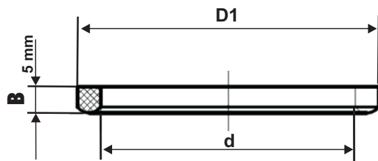
nákres těsnění
