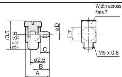
M-5ALHN-4 M-5ALHU-3/-4
